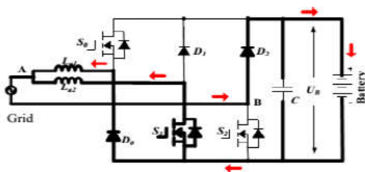
(d) Grid charging state 4 (Ugrid<0)
