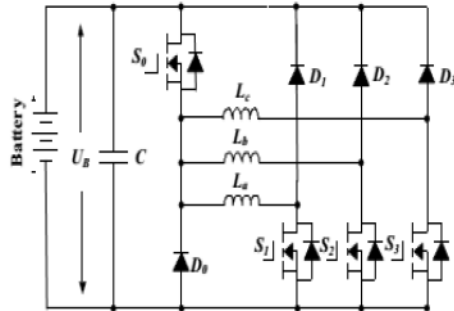
(d) Operation circuit under mode 4
