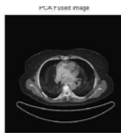
Figure3:PCA Output
