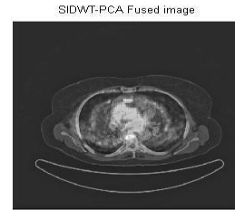
Figure7:SIDWT-PCA
